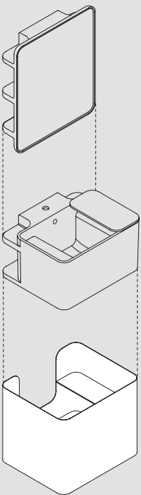
59,5x49,5xH50,5 cm ANF CES € 380,00
