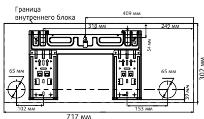
SYSPLIT WALL SMART 09 V2 HP Q 2021 год
