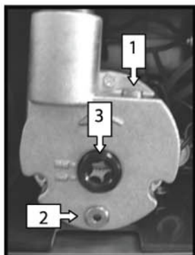
Вид сзади MINI JUMBO (задняя панель снята)
