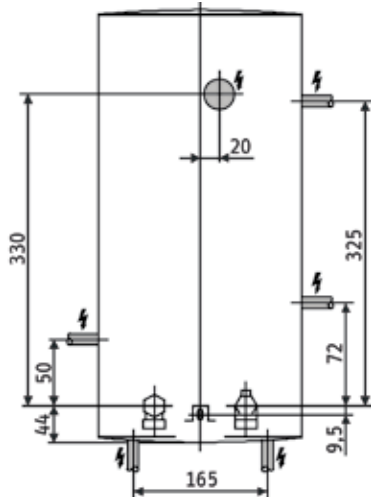
Maße für Elektroanschluss oben und aufputz (AP)
