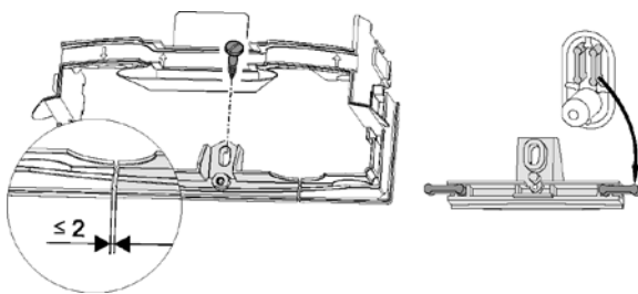
Montage mit geteiltem Unterteil
