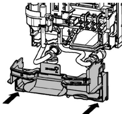
Montar y enclavar la parte inferior del panel trasero
