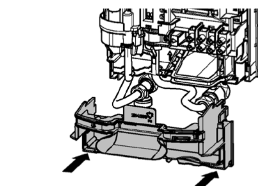
Монтаж и фиксация нижней части задней панели
