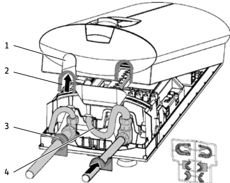
Montagehinweise für AP-Armaturen
