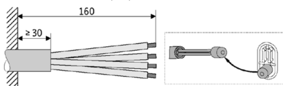
Подготовка кабелей электропроводки
