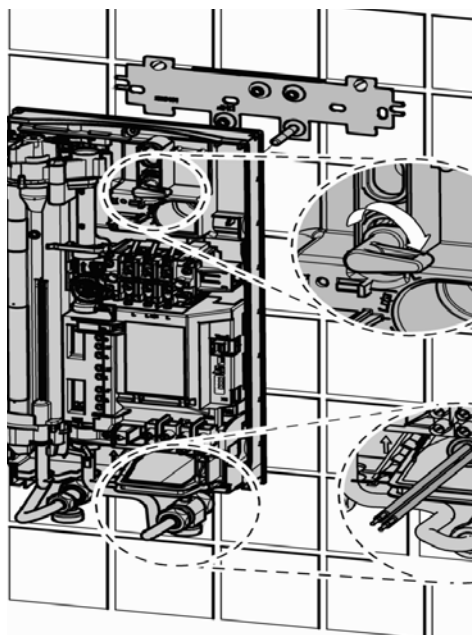
Zavěšení přístroje
