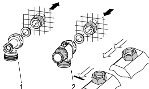
Подвод воды
