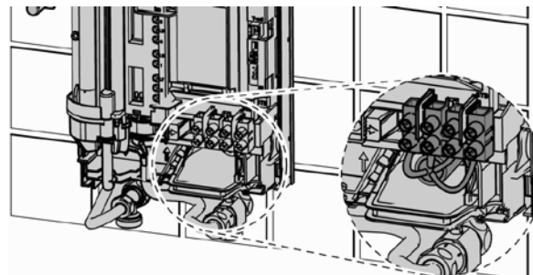
Acometida eléctrica
