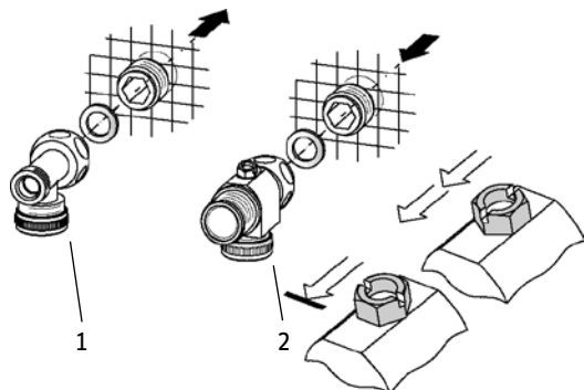
Wasseranschluss
