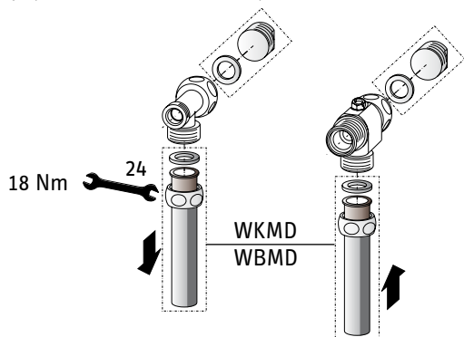
Připojení armatur instalovaných na stěně
