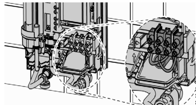
Электрическое соединение
