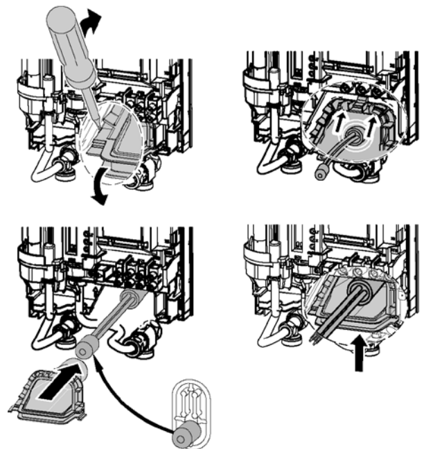
Demontage und Montage Kabeltülle
