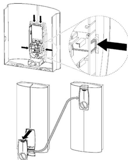
Gerätekappe bei Untertisch-Montage
