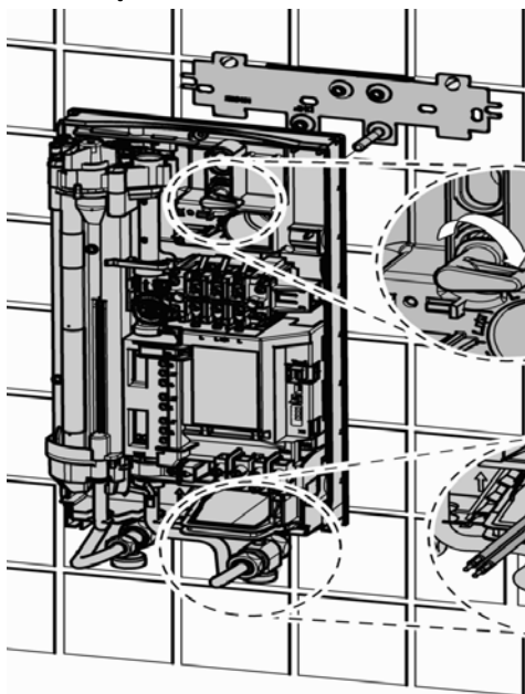
Zawieszenie urządzenia
