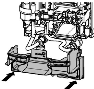
Montáž a zajištění spodní části zadní stěny
