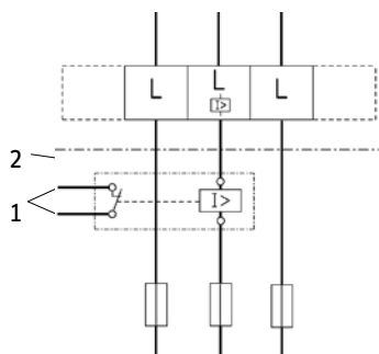
Předřazený spínač s LR 1-A
