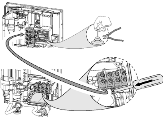
Elektroanschluss oben
