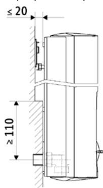
Wymiary montażowe przy instalacji na płytkach ceramicznych
