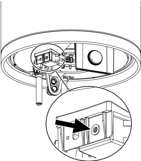
Bouton de réarmement du limiteur de sécurité
