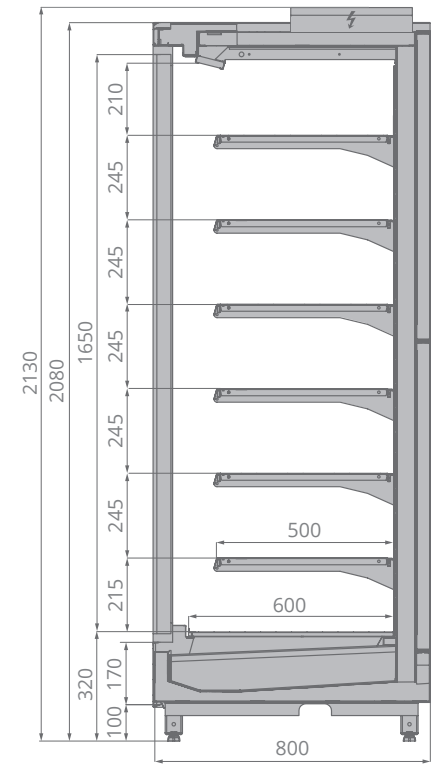
TESEY SLIM ESC
