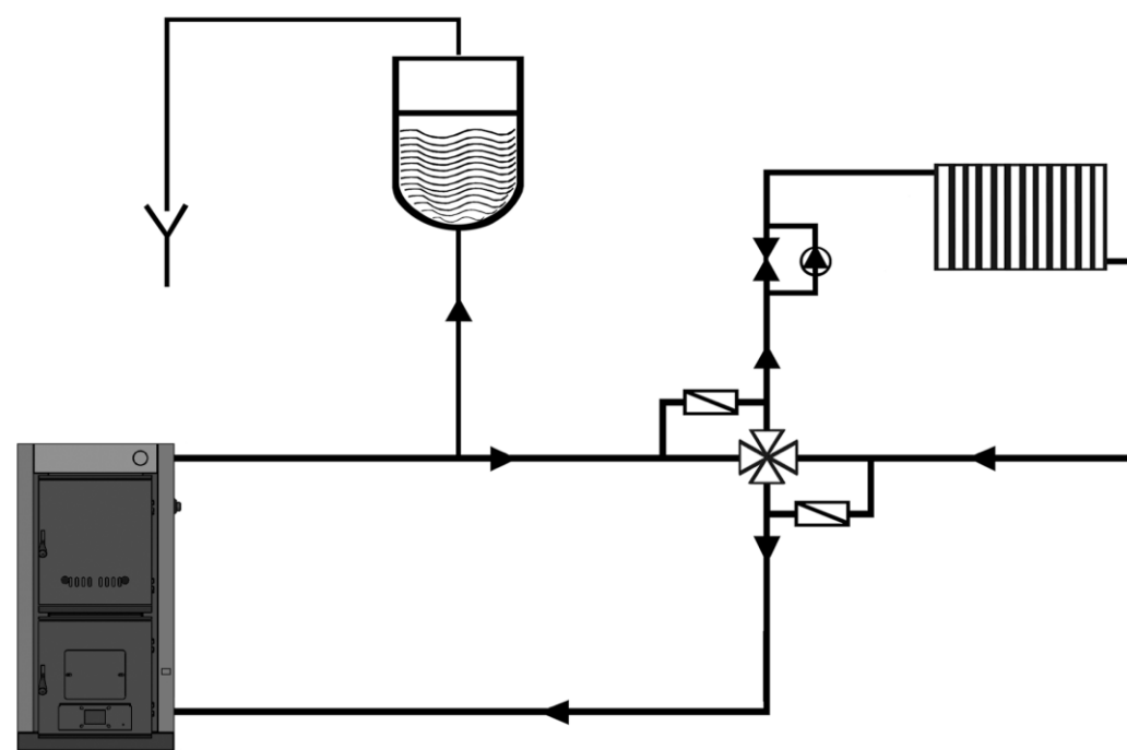
Рис.14 Без теплоаккумулятора
