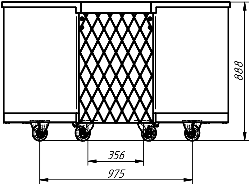
Вариант с поворотными колесами
