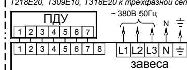
Схема подключения T206E10, T209E10, T212E20, T218E20, T309E10, T318E20 к трёхфазной сети и ПДУ.
