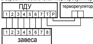
2-й вариант подключения терморегулятора
