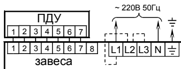
Схема подключения T206E10 к однофазной сети и ПДУ.
