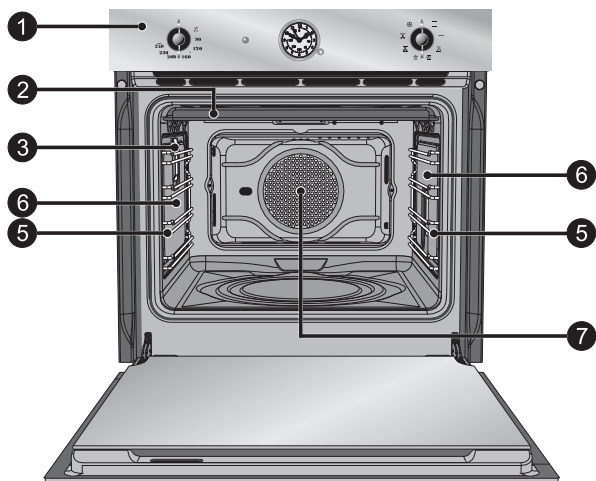
Многофункциональная модель
