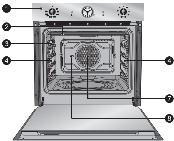
Пиролитическая модель
