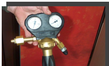
Манометры давления
